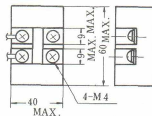
注3. 二点鎖線で示した2種類の外形のものとあります。
