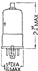
1H5GT
