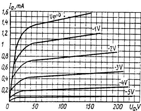
Усредненные анодные характеристики U_t = 1,2 V, U_{g2} = 45 V, U_{g3} = 0 V Average anode characteristics U_t = 1.2 V, U_{g2} = 45 V, U_{g3} = 0 V
