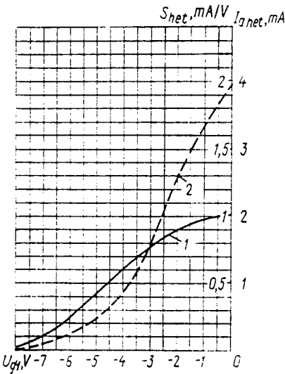
Усредненные характеристики гетеродина (сетки вторая и четвертая соединены с анодом): 1 — крутизна; 2 — анодно-сеточная U_t = 1,2 V, U_a = U_{g2} = 45 V Averaged characteristics of heterodyne oscillator (grid 2 and grid 4 are connected with anode): 1 — transconductance; 2 — anode-grid U_t = 1.2 V, U_a = U_{g2} = 45 V
