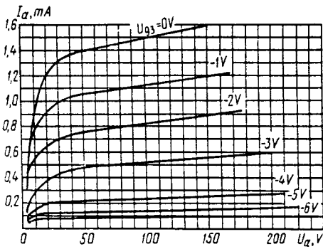
Усредненные анодные характеристики U_t = 1,2 V, U_{g2} = 45 V, U_{g1} = 0 V Averaged anode characteristics U_t = 1.2 V, U_{g2} = 45 V, U_{g1} = 0 V
