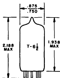
SMALL BUTTON BASE 9 PIN JEDEC E9-1
