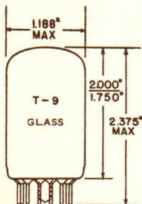
BASE 12 PIN BUTTON JEDEC E12-70
