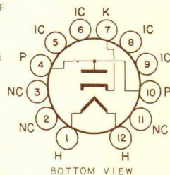
BASING DIAGRAM JEDEC 12BL
