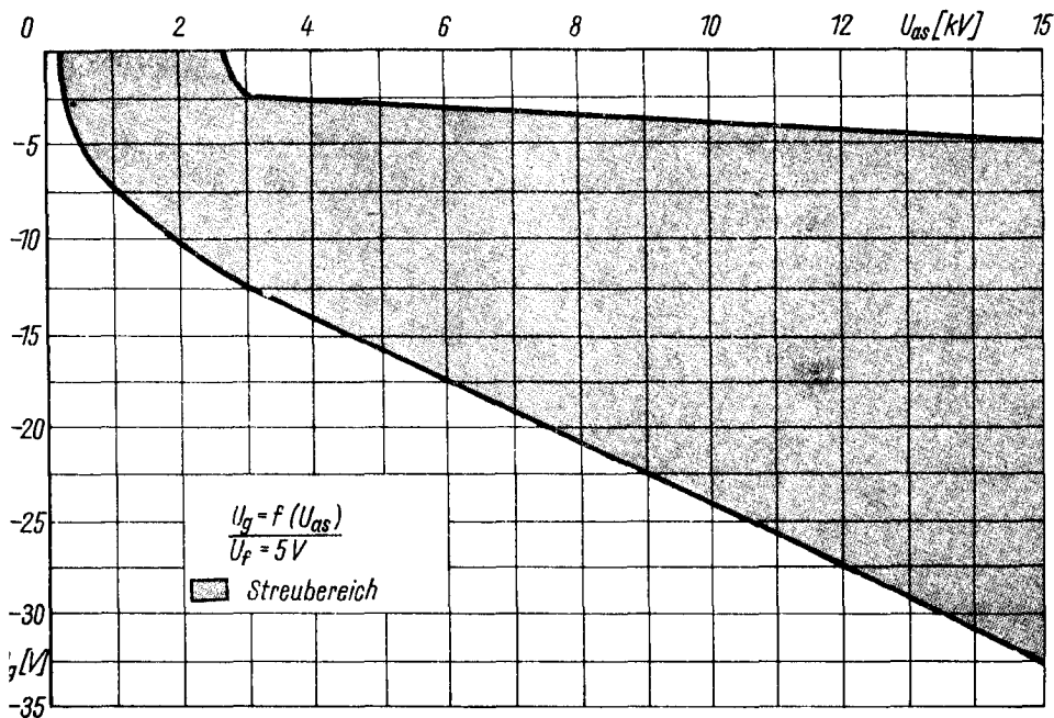
Zündkennlinien-Streubereich
