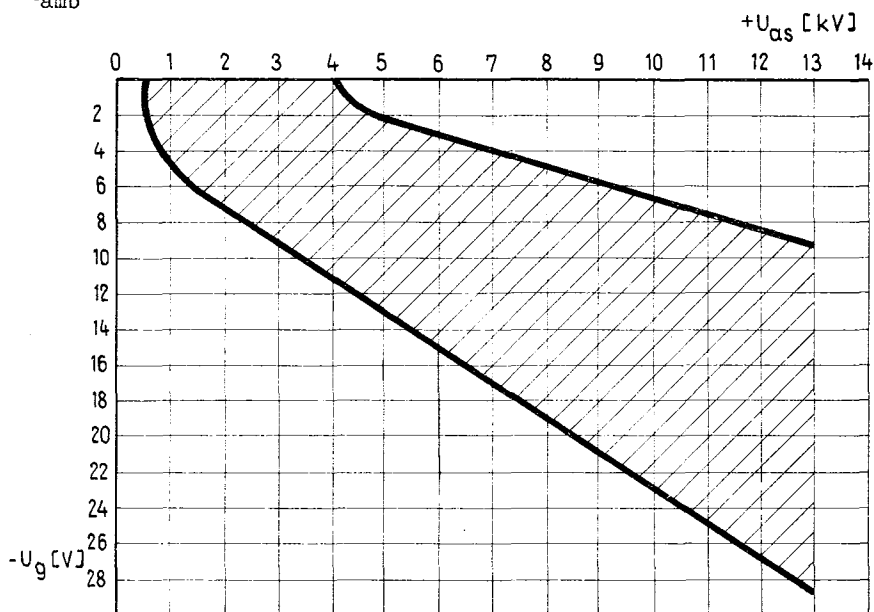
Zündkennlinien-Streubereich
