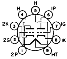
BOTTOM VIEW MINIATURE BUTT 9 PIN BASE 9A
