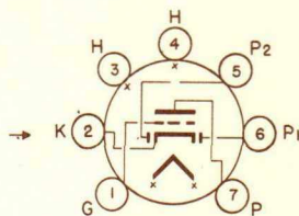
BOTTOM VIEW BASING DIAGRAM JEDEC 7BT
