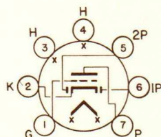
BOTTOM VIEW BASING DIAGRAM JEDEC 7BT
